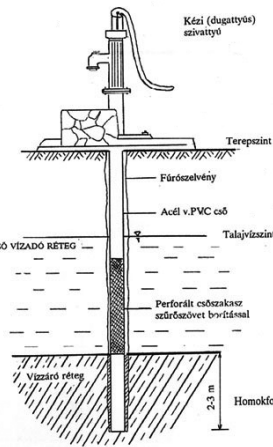
Talajvízre telepített fúrt kút Gerecsér Á. nyomán [1.]
